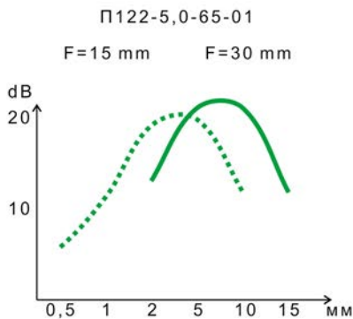
ГРАФИКИ РЕАЛЬНОГО ЗАПАСА ЧУВСТВИТЕЛЬНОСТИ (ОБРАЗЕЦ МД 2-0-1)
