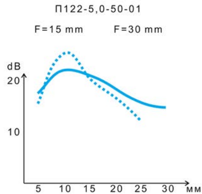
ГРАФИКИ РЕАЛЬНОГО ЗАПАСА ЧУВСТВИТЕЛЬНОСТИ (ОБРАЗЕЦ МД 2-0-1)
